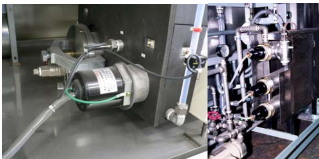
写真1 取付例
