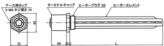
図2 GK5・GA5型（標準キャップ仕様）
