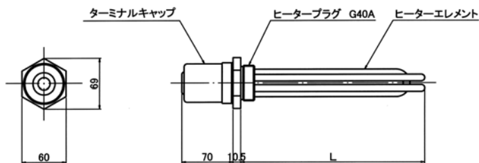
図1 GA4型（標準キャップ仕様）
