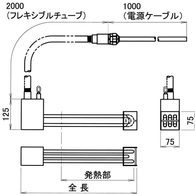
図1 ステンレスモールド潜水ヒーター
