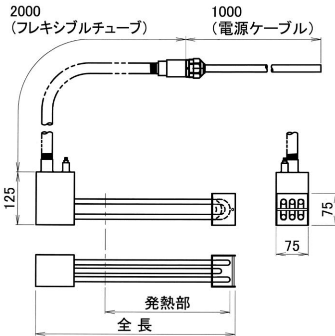
図1 ステンレスモール潜水ヒーター
