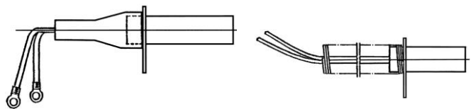
図2 ツバ付防水型
