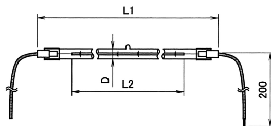
図1 ハロゲンヒーター
