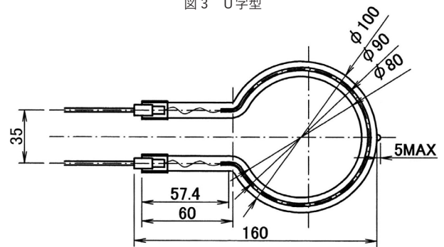
図4 リング型
