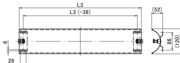
図2 反射笠
