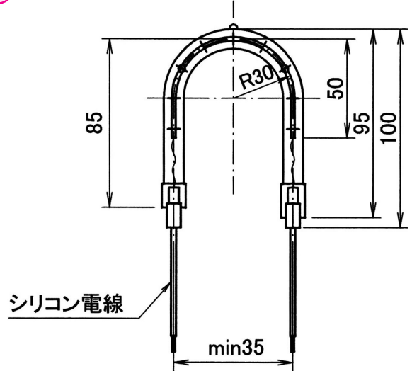
図3 U字型
